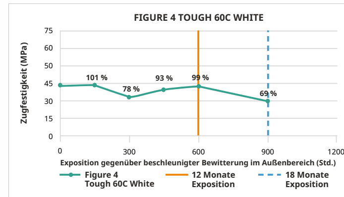
Zugfestigkeit im Außenbereich
