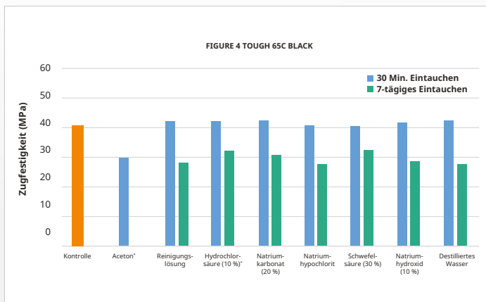
Chemische Zugfestigkeit
