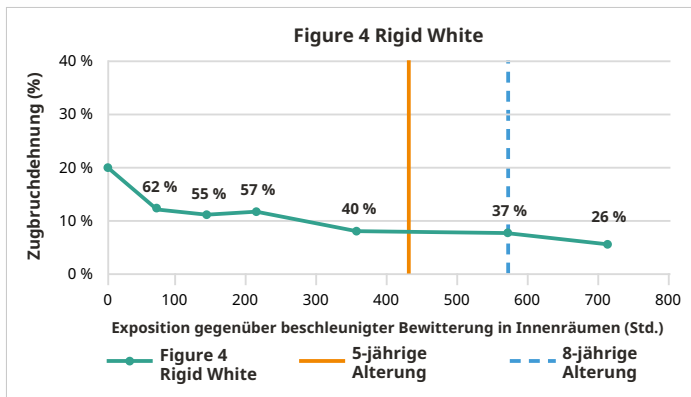
Dehnung in Innenräumen
