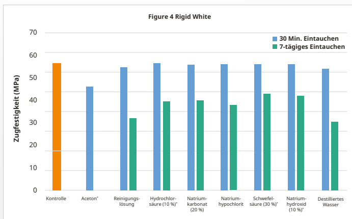
Chemische Zugfestigkeit
