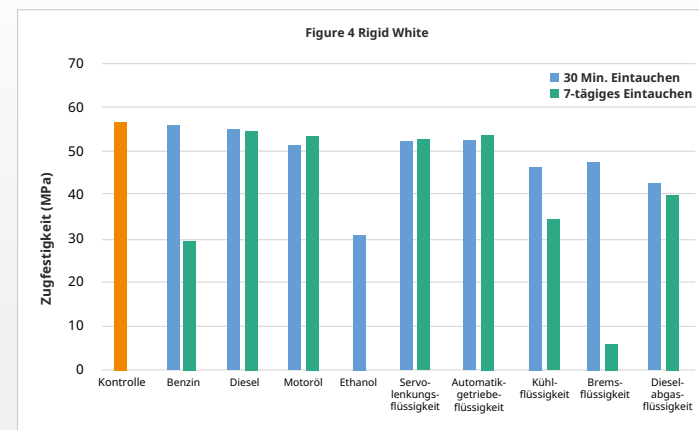
Zugfestigkeit bei Kfz-Flüssigkeiten
